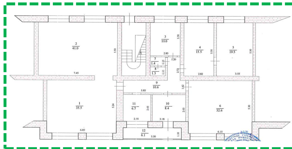
Технический паспорт - Поэтажный план здания 1 этаж
